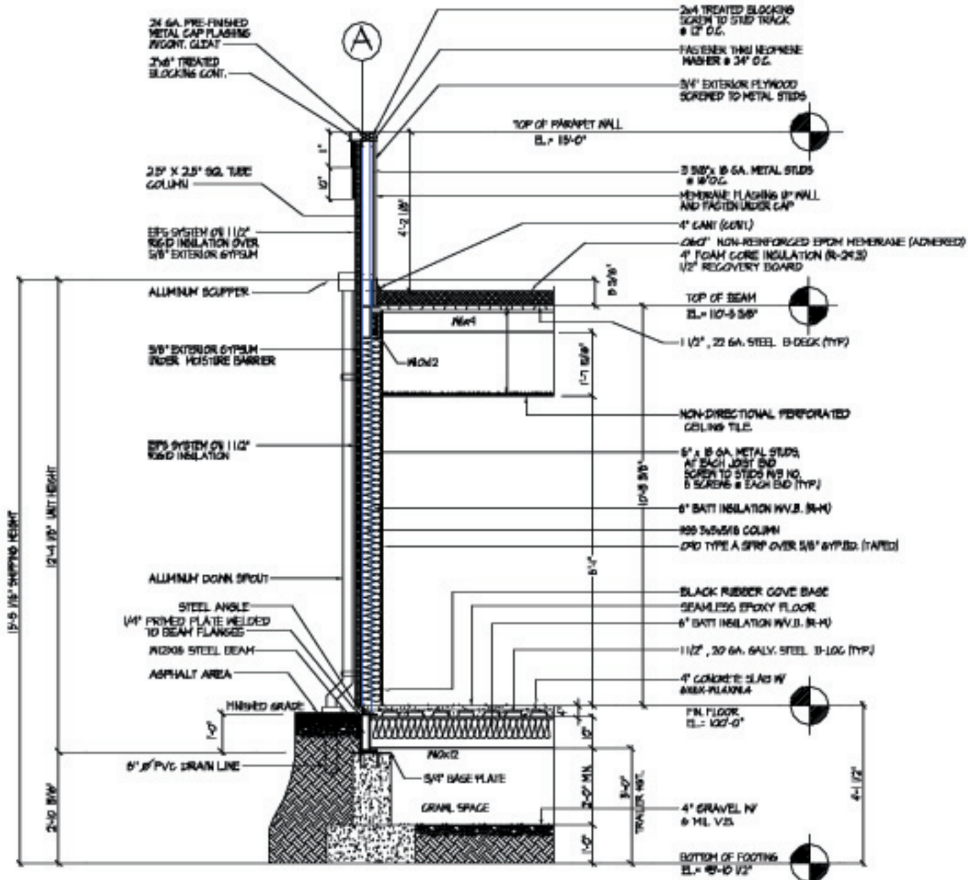
SECTION I SCALE: 1/2" = 1'-0"
